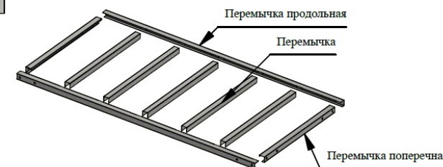
Полка-решетка
